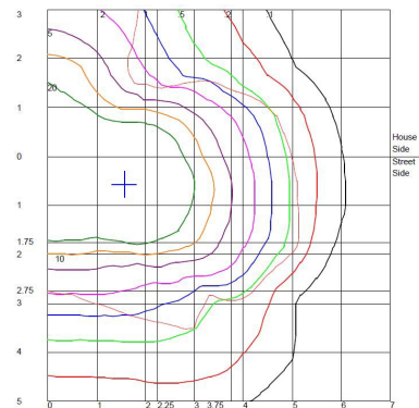
Isolux
