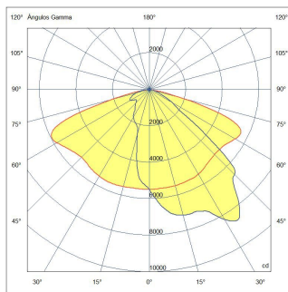
Curva Polar
